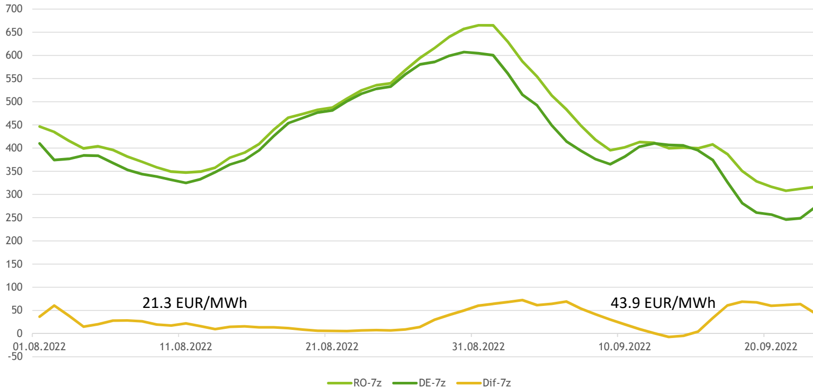
Preturi PZU Romania / Germania - media la 7 zile - EUR/MWh
